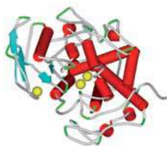
Рис. 5. Пространственная структура тирозиназы – фермента, необходимого для синтеза меланина (PDB 1WX3) (сферы желтого цвета – атомы меди в активном центре фермента)
